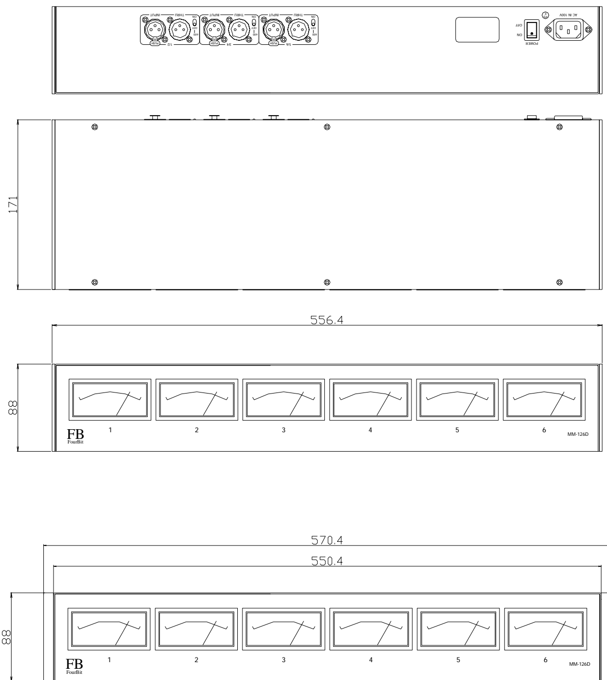
オプション(別売) 木製サイドパネル装着時
