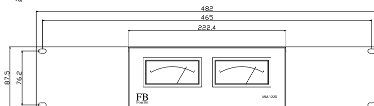
オプション(別売) ラックマウントアングル装着時
