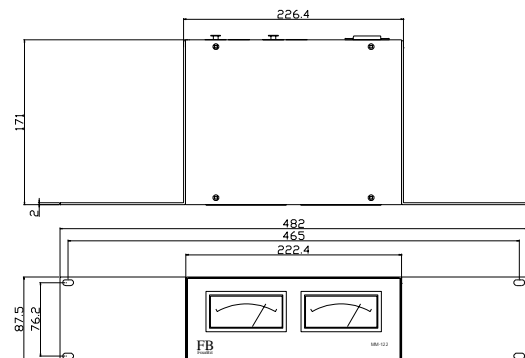
オプション(別売) ラックマウントアングル装着時
